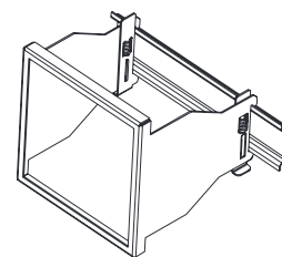
Adapter ATS1 ( 92^{+0.8} \times 92^{+0.8} mm)
