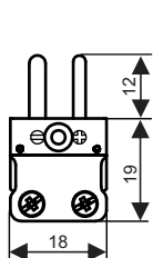
Mini konektor
