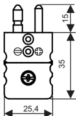
Standardni konektor
